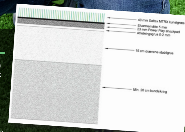
Sådan er kunstgræsbanen på JYSK park bygget op. Illustration: Winther Sport & Fritid
